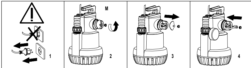
Montaje del flotador / Float assembly / Montage du flotteur / Schwimmernontage / Montaggio del galleggiante / Montagem do bóia / Montage van de vlotter
