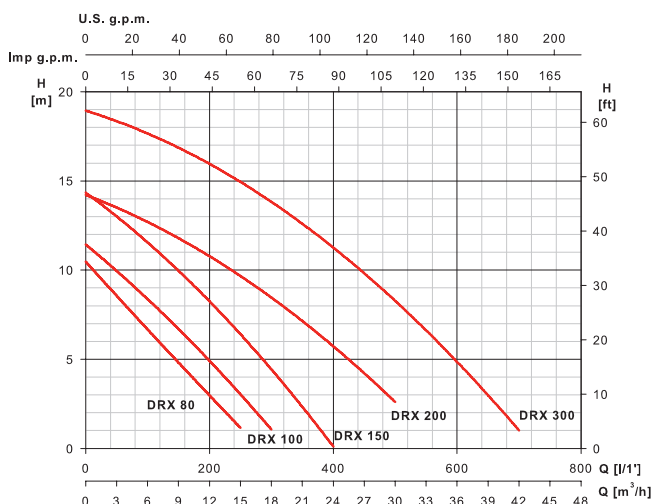
Curve di prestazione a 2900 rpm
